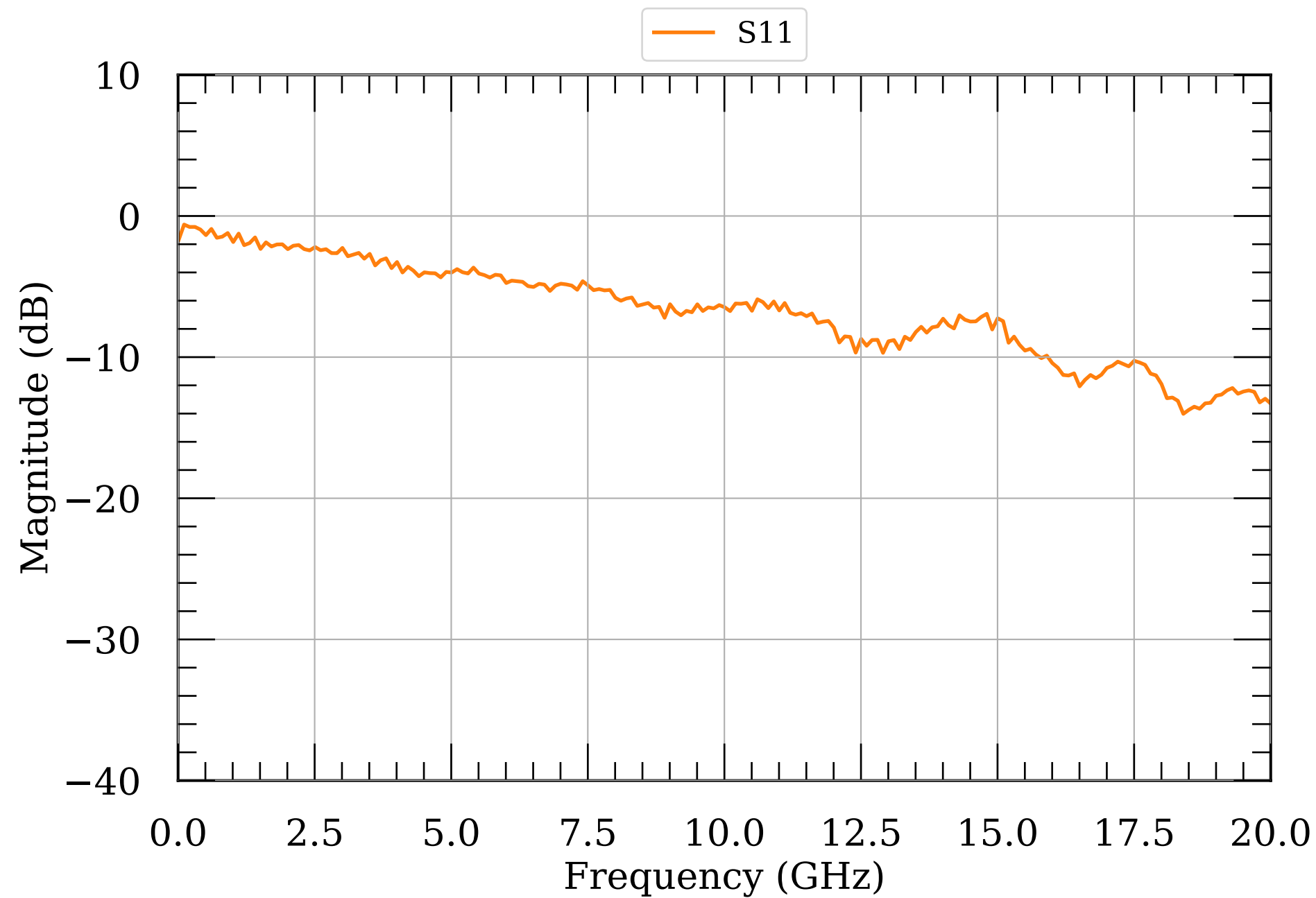
LNA S-params module027
